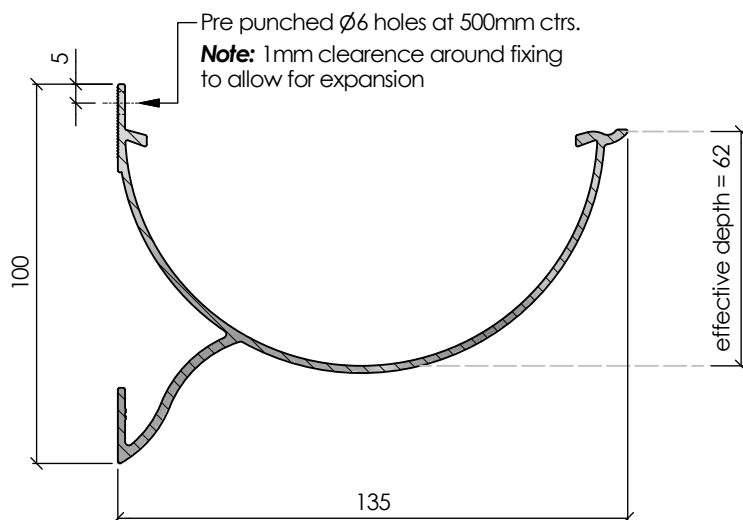
Section A-A (1 : 2)
