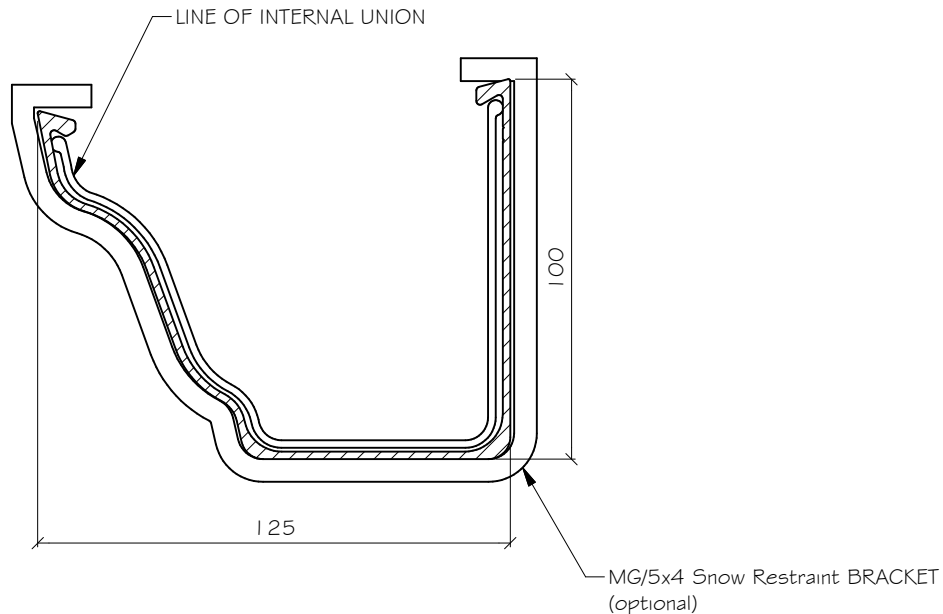
SECTION A-A ( 1 : 2 )
